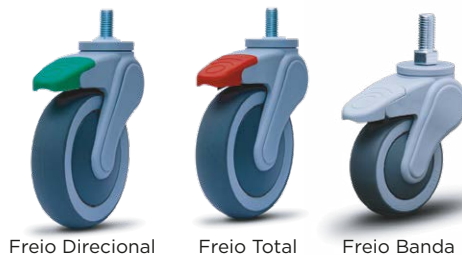
Freio Direcional Freio Total Freio Banda
